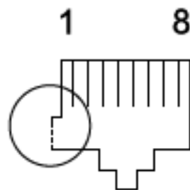
8P8C
